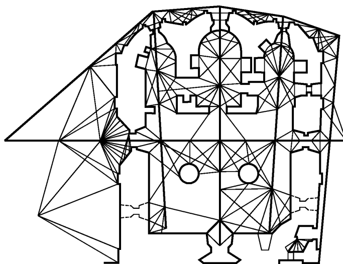
Рисунок Б.2 — Схема обмера плана с причалками
